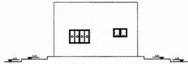
1 FACHADA LATERAL ESCALA 1:50
