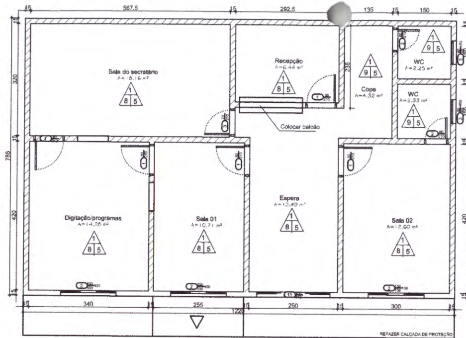
1 PLANTA BAIXA
