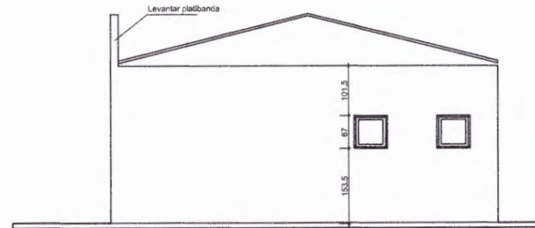
FACHADA LATERAL
