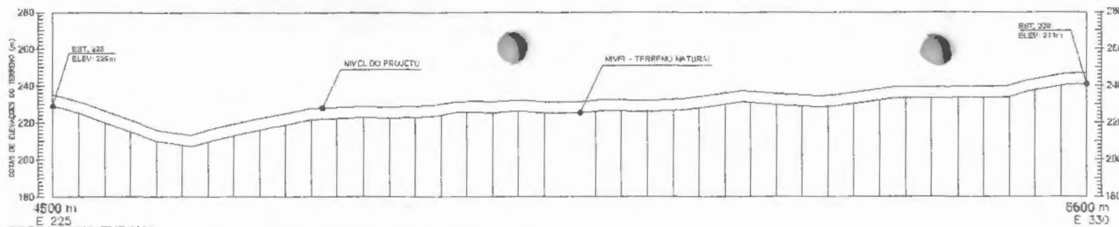
PERFIL LONGITUDINAL EST. 225 A EST. 330
