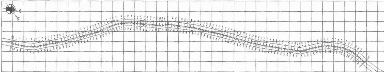
PLANTA DE ESTAQUEAMENTO TRECHO ANJICO - (PARTE 2) - EST. 110 A EST. 225 PXT, (m) 0,303,00m
