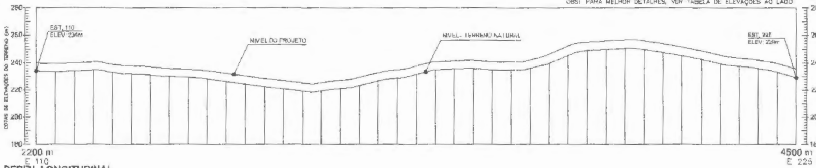
PERFIL LONGITUDINAL EST. 110 A EST. 225
