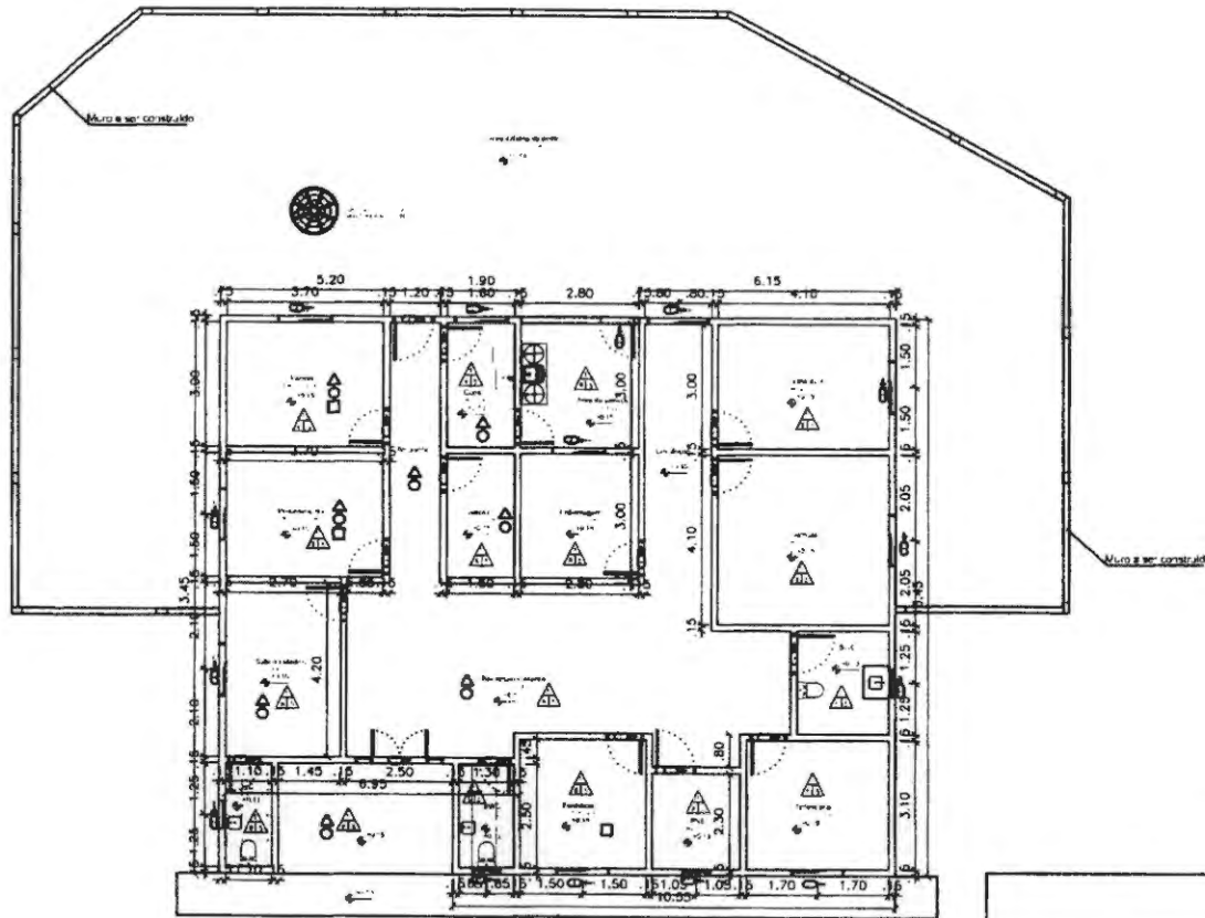
PLANTA BAIXA ESCALA: 1/50
