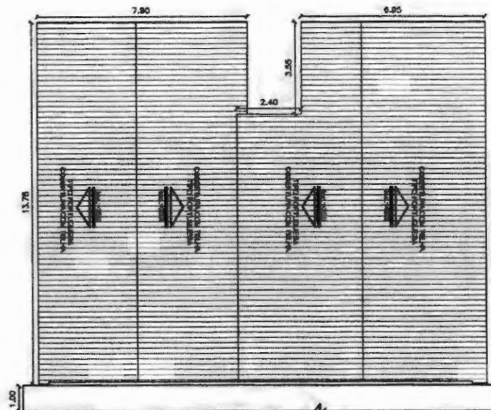
PLANTA DE COBERTURA ESCALA: 1/75
